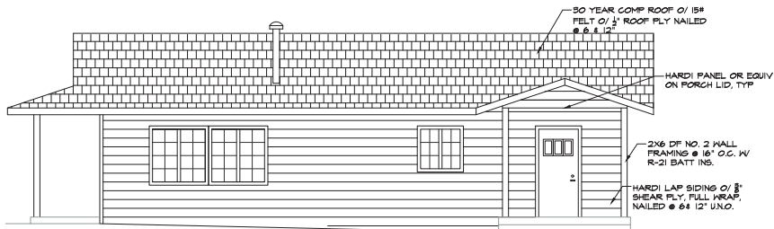
RIGHT ELEVATION
